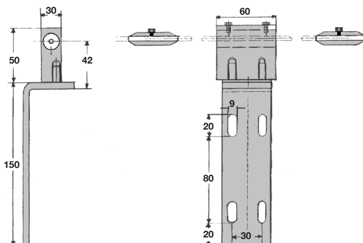
Attacco per portone a due ante asimmetriche cod. 700476X
