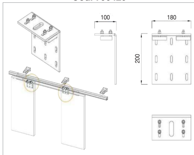
Attacco cinghia porta per seconda anta Cod. 790420
