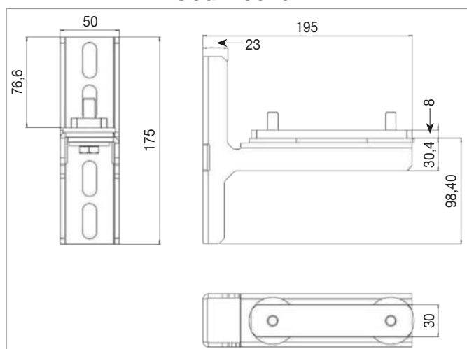
Mensola parete forati o carton gesso Cod. 790404
