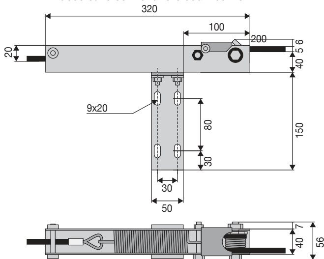
Attacco cavo con tenditore cod. 700478
