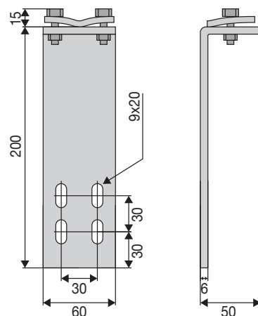
Attacco cavo per seconda anta cod. 700476
