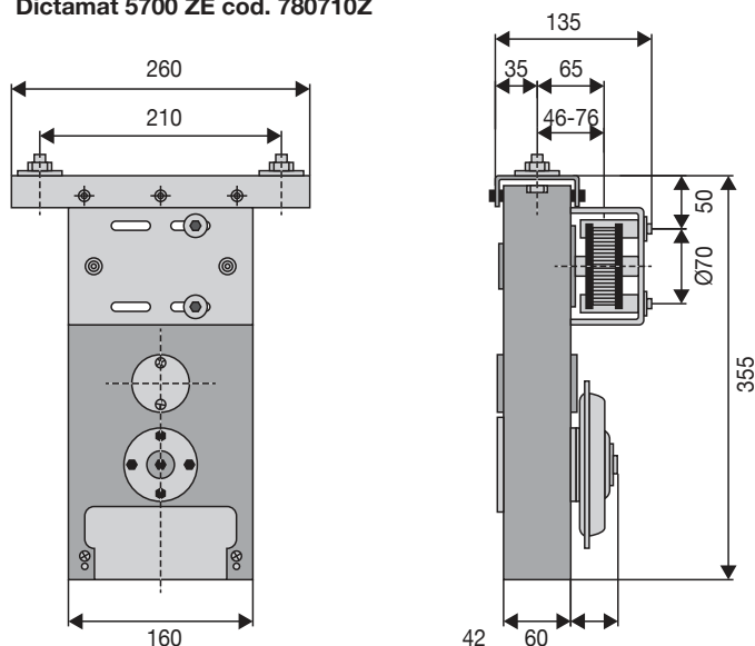
Dictamat 5700 ZE cod. 780710Z
