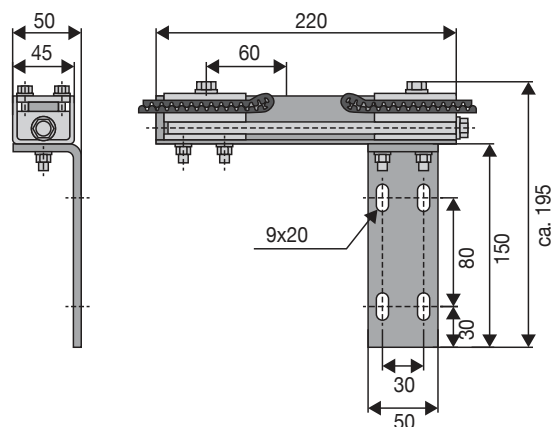
Attacco cinghia con tenditore cod. 710497
