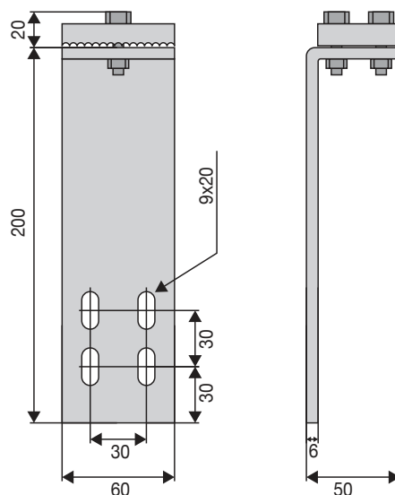
Attacco cinghia con tenditore cod. 710497
