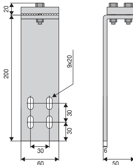
Attacco cinghia con tenditore cod. 710497
