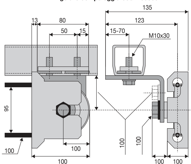
Angolare con puleggia cod. 700530
