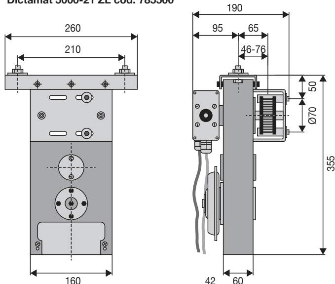
Dictamat 5000-21 ZL cod. 785500
