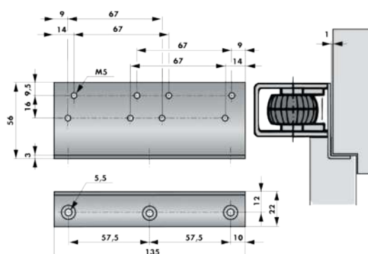
Codice 205220
