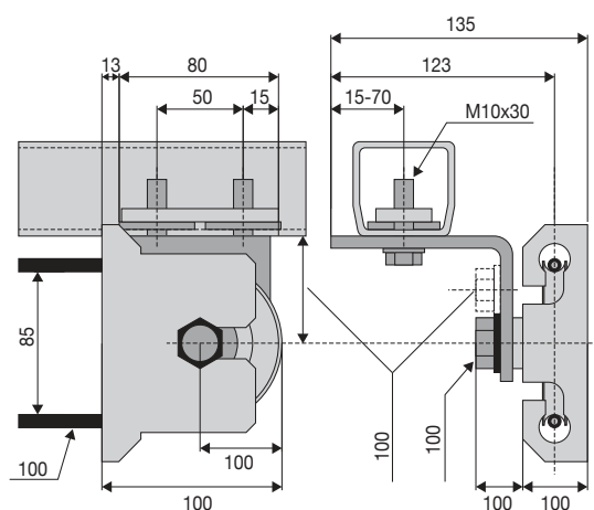
Angolare con puleggia cod. 700530
