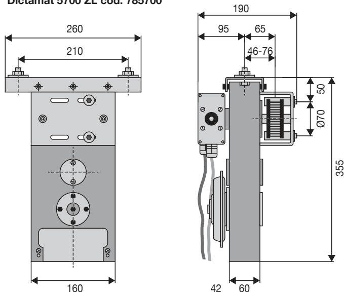
Dictamat 5700 ZL cod. 785700
