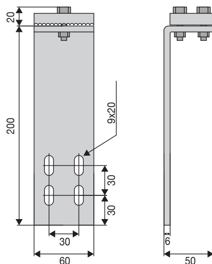
Attacco cinghia per seconda anta cod. 710495
