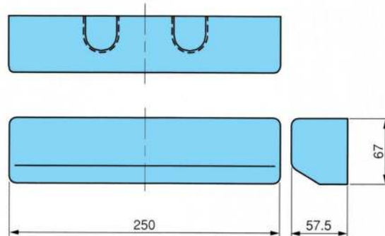
COPERTURA (CARTER)
