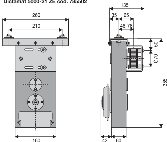
Dictamat 5000-21 ZE cod. 785502
