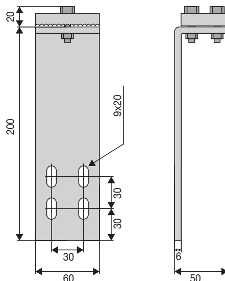
Attacco cinghia per seconda anta cod. 710495
