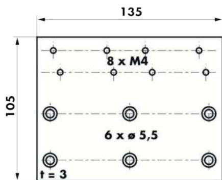
Codice 205279
