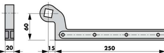
Cerniera inferiore cod. 460086-300 (300 kg) 460086-600 (600 kg)
