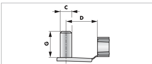
Attacco a incastro sullo stelo con perno per forcina
