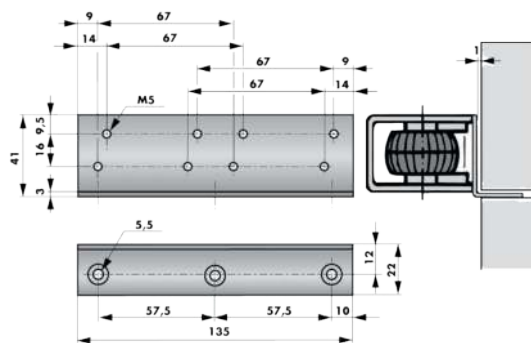
Codice 205221
