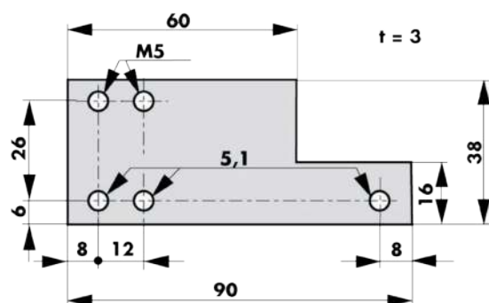
Codice 205256
