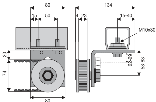
Angolare con puleggia cod. 710492
