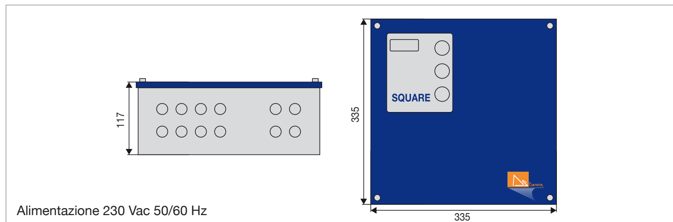
Dictamat 5700 ZE cod. 780710Z
