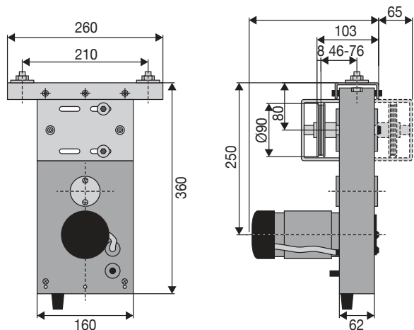
Dictamat 3700 SE cod. 730072/M
