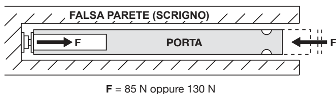
Assorbimento urto
