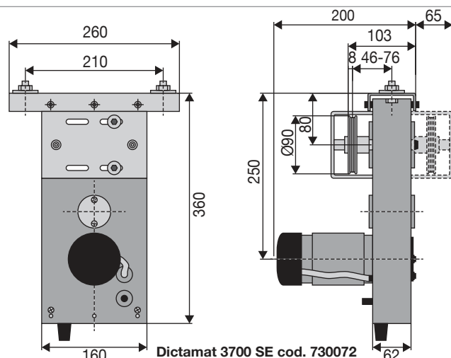
Dictamat 3700 SE cod. 730072
