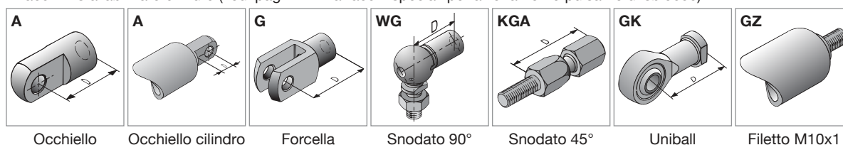
Occhiello Occhiello cilindro Forcella Snodato 90° Snodato 45° Uniball Filetto M10x1
