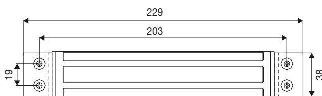
Elettromagnete cod. 040281SET
