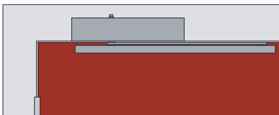
COU 52/53 R - Su architrave del telaio
